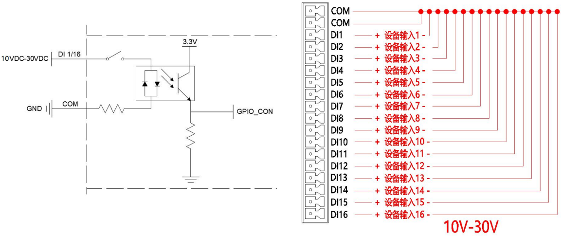
NPN模式
