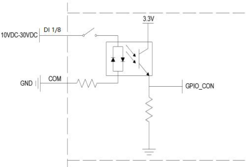
DI引脚的接线图：
