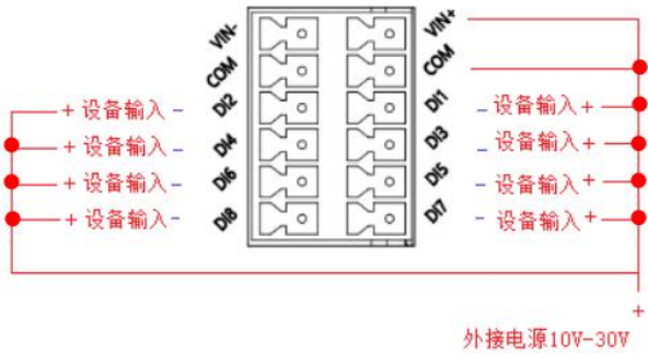
PNP 模式
