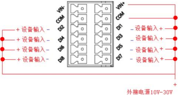
PNP模式
