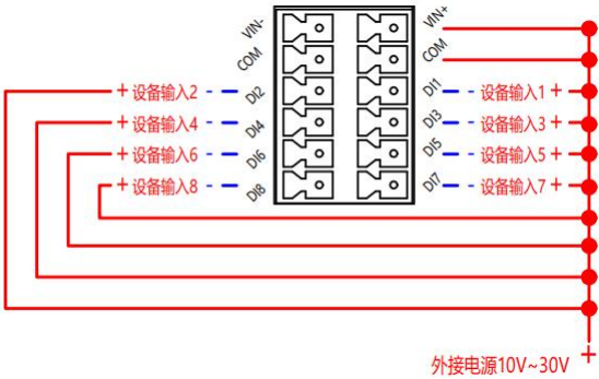
PNP模式
