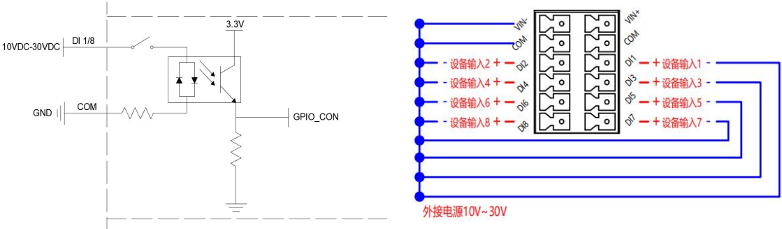
NPN模式
